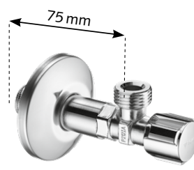
Eckventil mit Regulierfunktion mit Halbzollgewinde und COMFORT-Griff
