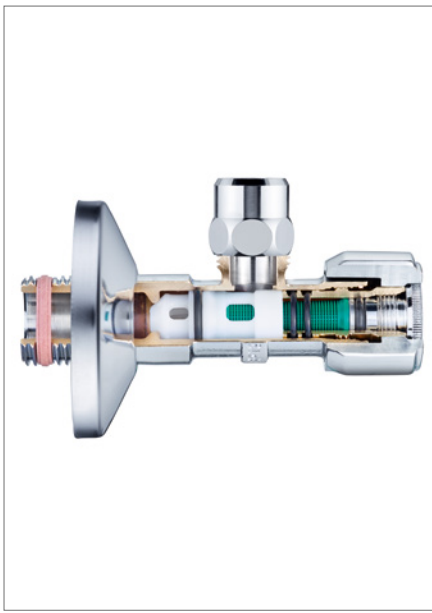
Eckventil mit Regulierfunktion mit Filter
