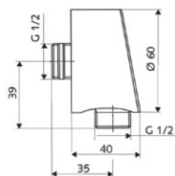
SCHELL nástenné pripojovacie koleno PURIS Designové vyhotovenie prívod 1/2" / DN 15, vývod 1/2" / DN 15
