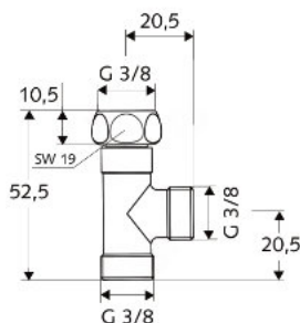
SCHELL T-kus 3/8" x 3/8" x 3/8" / DN 10 s jednou prevlečnou maticou 3/8"
