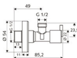
SCHELL rohový regulačný ventil PINT s designovou rukoväťou 1/2" x 1/2"
