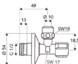
SCHELL rohový regulačný ventil COMFORT Regulačný ventil s dvojitou spätnou klapkou prívod 1/2" / DN 15
