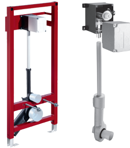
WC-module MONTUS/ Inbouw-W druckspoeler COMPACT II
